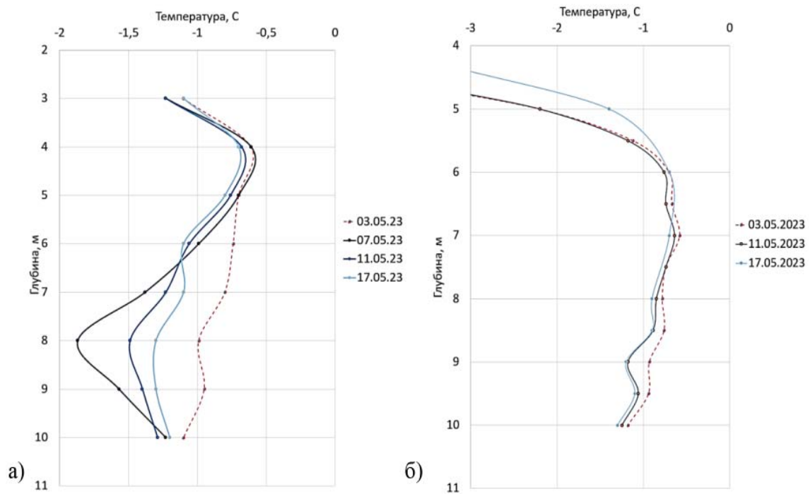
Рис. 6. Профили температуры грунта на расстоянии 750 мм от охлаждающей скважины (а) и на расстоянии 1500 мм от охлаждающей скважины (б)
