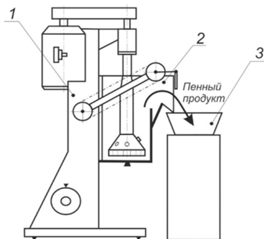
Рис. 1. Экспериментальный стенд:
