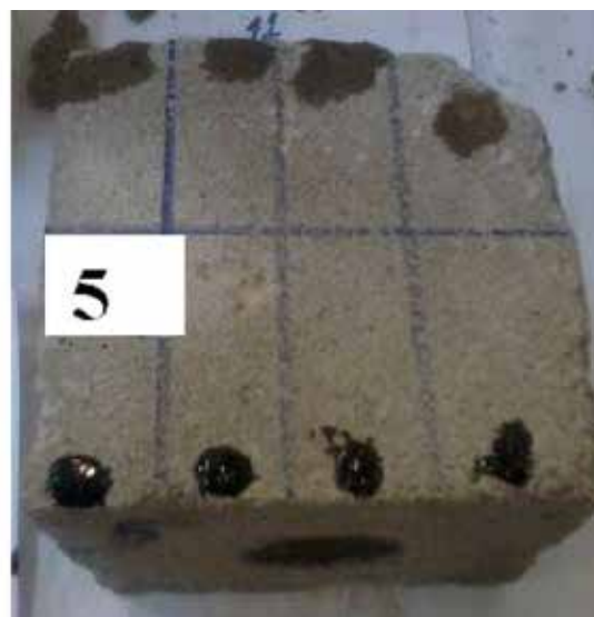
Рис. 1. Характер распространения нефтяного пятна на поверхности визуально плотного и пористого бетона (блоки 2 и 5)
