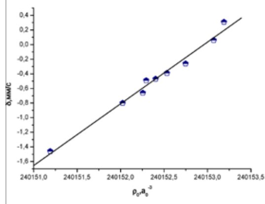
Рис. 4. Зависимость между экспериментальным изомерным сдвигом и рассчитанной методом BP86/TZ2P+ электронной плотностью на ядре ^{127}\text{I}
