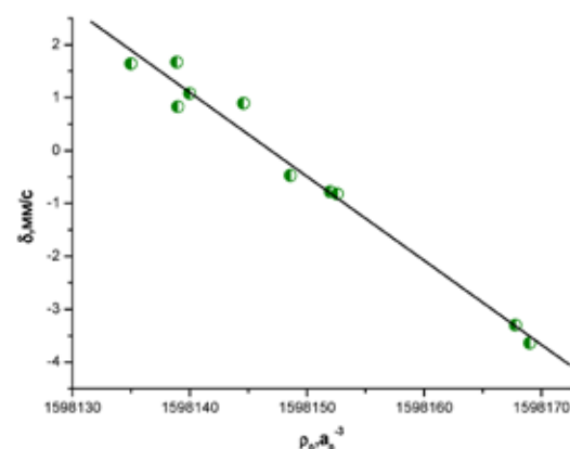
Рис. 8. Зависимость между экспериментальным изомерным сдвигом и рассчитанной методом BP86/TZ2P+ электронной плотностью на ядре ^{187}\text{Os}
