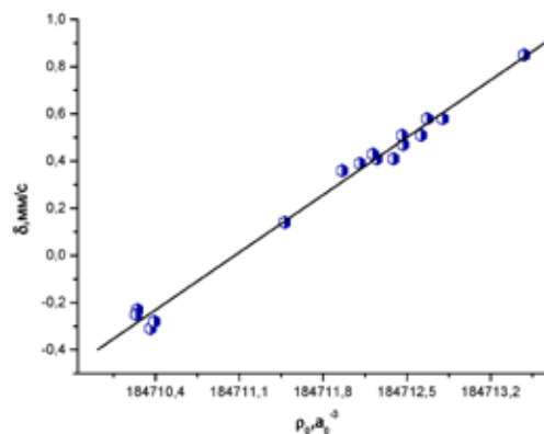
Рис. 2. Зависимость между экспериментальным изомерным сдвигом и рассчитанной методом BP86/TZ2P+ электронной плотностью на ядре ^{119}\text{Sn}
