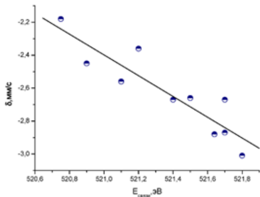
Рис. 11. Зависимость между экспериментальным изомерным сдвигом и рассчитанной методом BP86/TZ2P+ энергией связи в \text{SbCl}_5\text{L} комплексах
