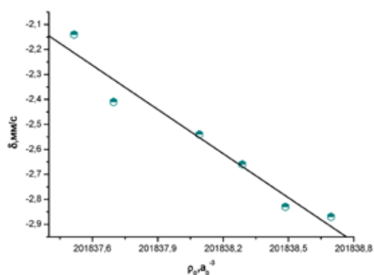
Рис. 5. Зависимость между экспериментальным изомерным сдвигом и рассчитанной методом BP86/TZ2P+ электронной плотностью на ядре ^{121}\text{Sb}
