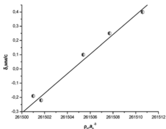
Рис. 3. Зависимость между экспериментальным изомерным сдвигом и рассчитанной методом BP86/TZ2P+ электронной плотностью на ядре ^{131}\text{Xe}
