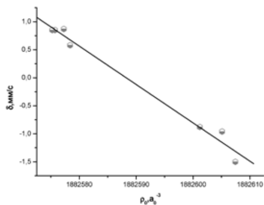
Рис. 6. Зависимость между экспериментальным изомерным сдвигом и рассчитанной методом BP86/TZ2P+ электронной плотностью на ядре ^{195}\text{Pt}
