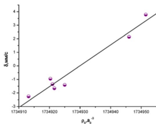
Рис. 5. Зависимость между экспериментальным изомерным сдвигом и рассчитанной методом BP86/TZ2P+ электронной плотностью на ядре ^{121}\text{Sb}
