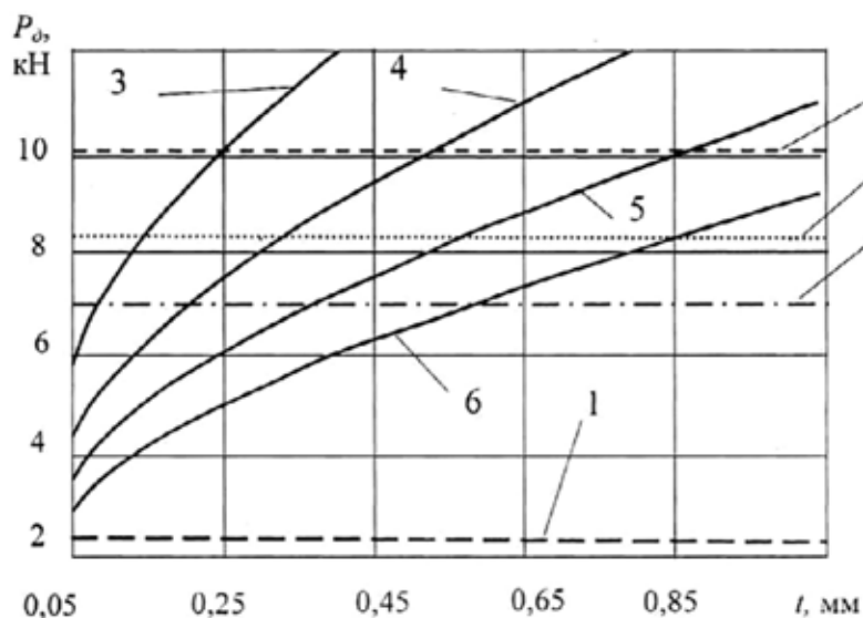
Рис. 3. Графики, определяющие допустимую область усилий деформирования на один ролик для заготовки диаметром 20 мм:
