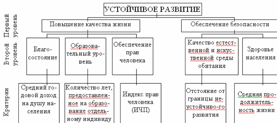
Рисунок 1. Система подцелей
